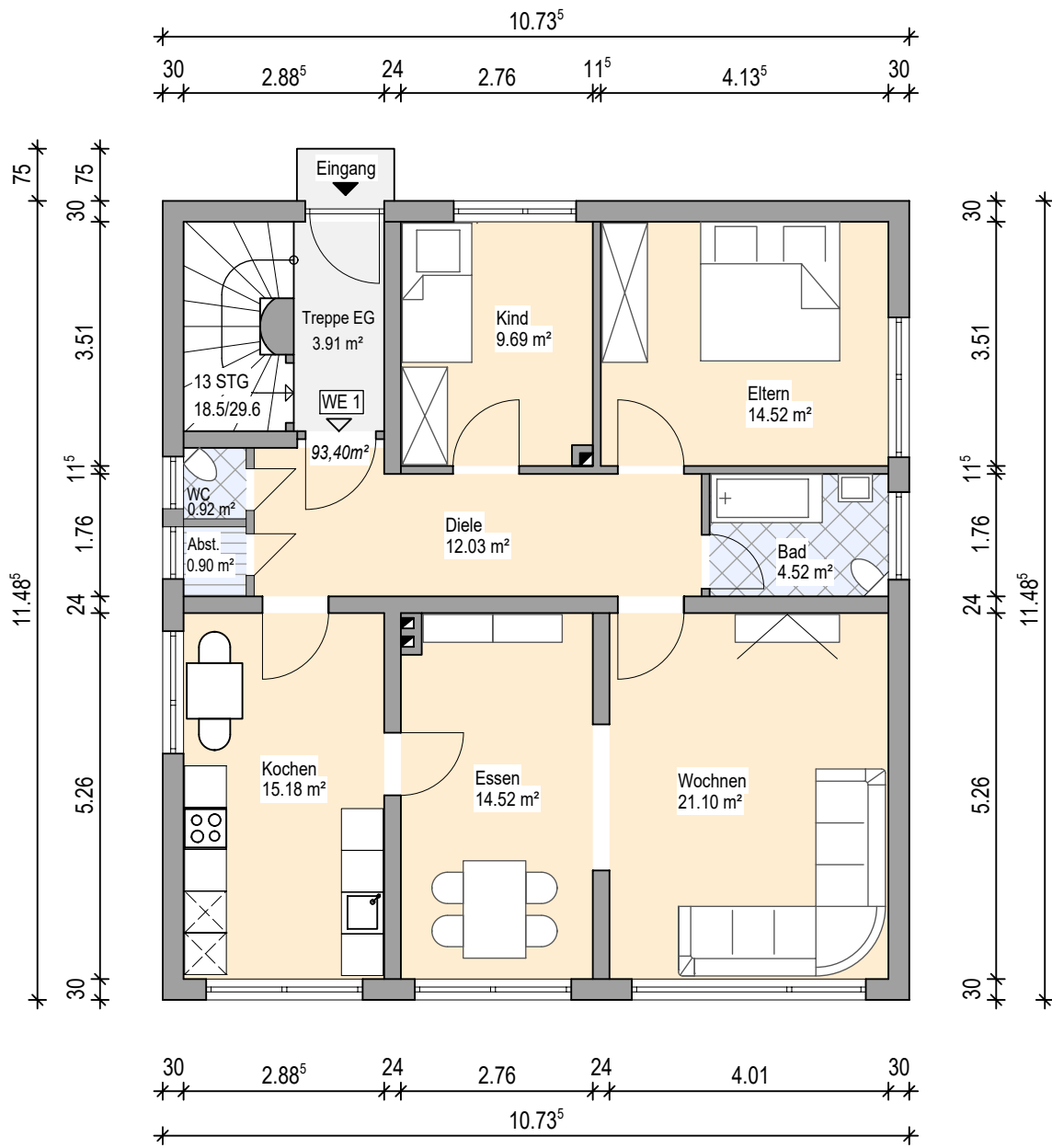
Erdgeschoss m 1 / 100
