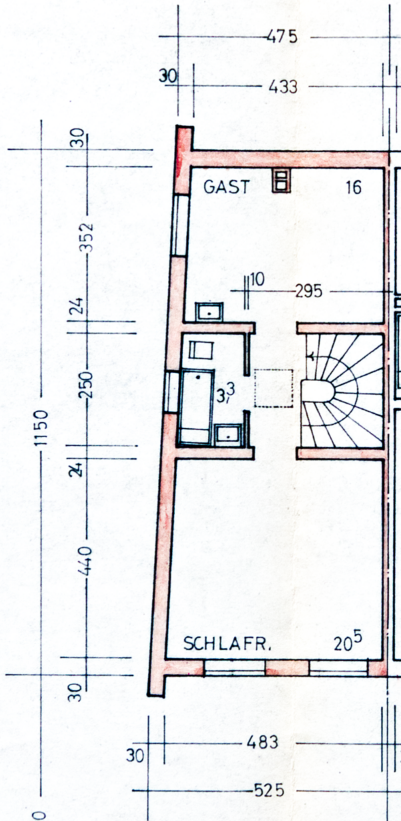
OBERGESCHOSS
