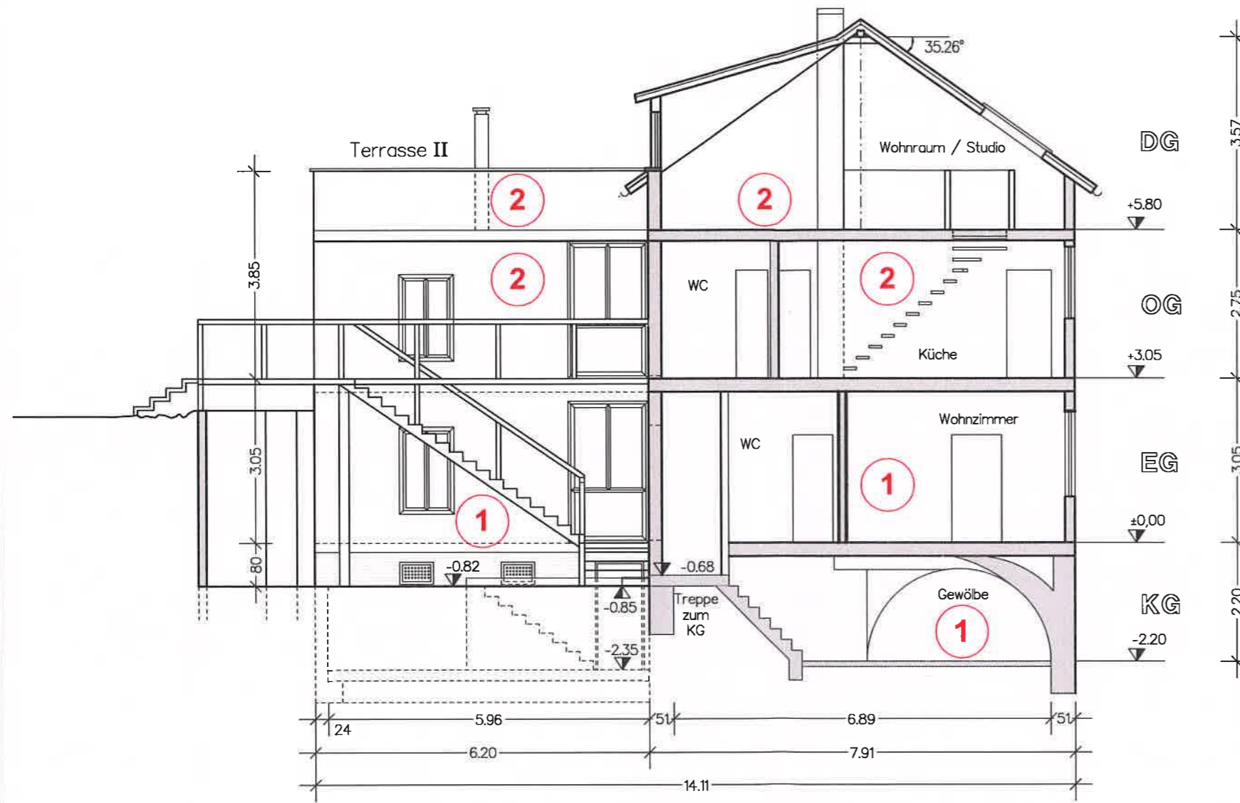
Schnitt A-A
