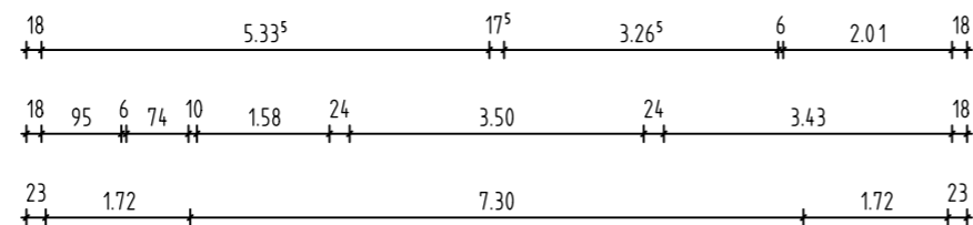
1.OBERGESCHOSS
