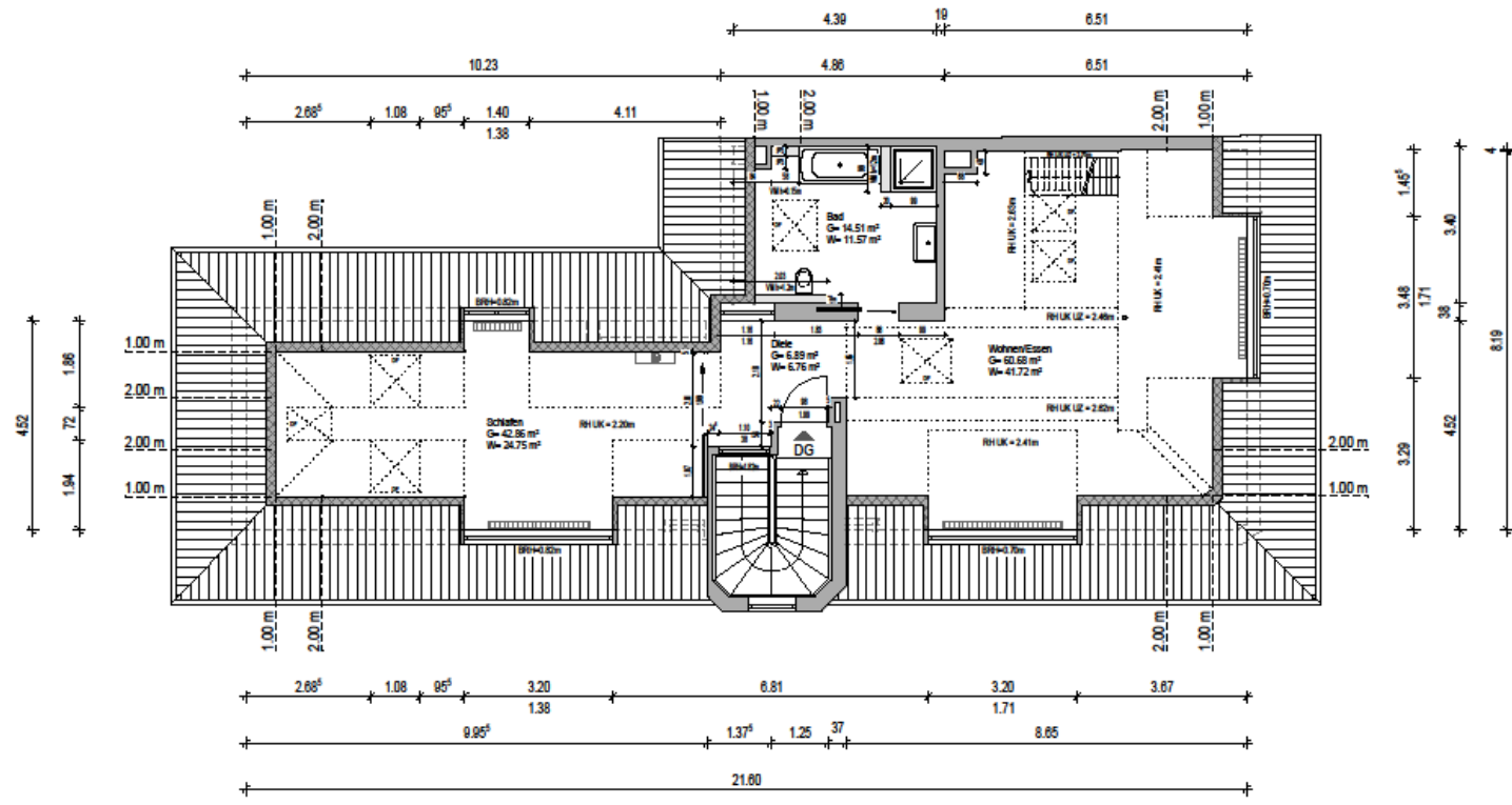
Grundriss Dachgeschoss M 1:100
